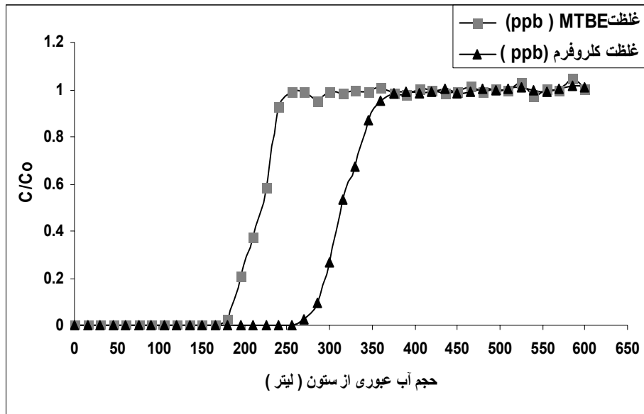
نمودار ۳ - منحنی شکست مربوط به تصفیه آب حاوی MTBE (100 ppb) ، کلروفرم (100 ppb) و کلر باقیمانده (0/2 ppm).
