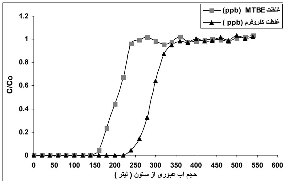
نمودار ۴ - منحنی شکست مربوط به تصفیه آب حاوی MTBE (100 ppb) ، کلروفرم (100 ppb) و کلر باقیمانده (0/5 ppm).
